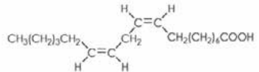
cis,cis -9,12-oktadekadienska kiselina
